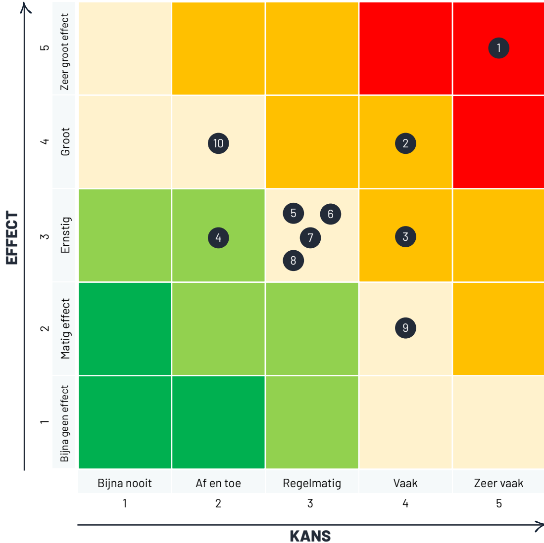
Figuur: Risicomodel
